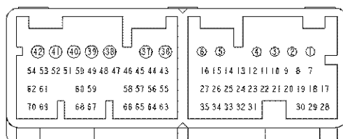
Fig.11 70 極回路番号
