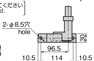
〔FA-1810-1B用フック・キーパー〕 Hook and keepers
