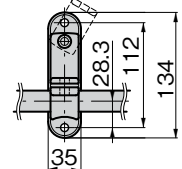
〔FA-1810-1A・1B用受け〕 catch
