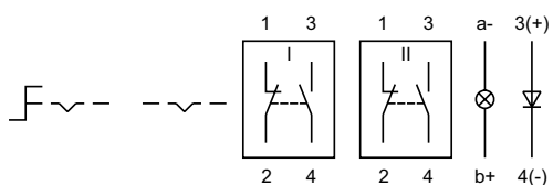
Wiring diagram 24
