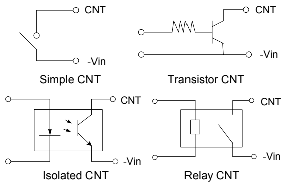
Fig. 71 CNT circuits
