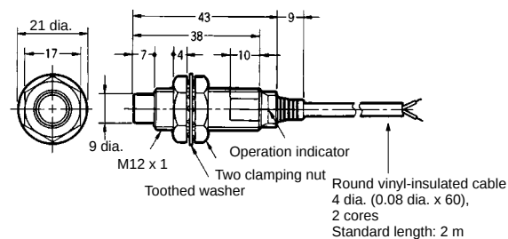
Fig. 11 : E2E-X5MY□
