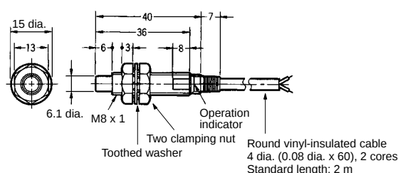
Fig. 9 : E2E-X8MD□ E2E-X5ME□/F□
