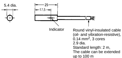
Fig. 3 : E2E-C1□□
