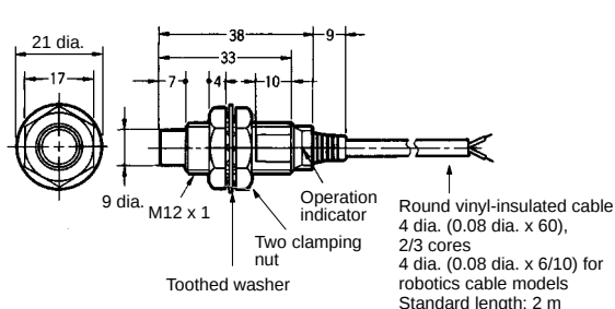
Fig. 9 : E2E-X8MD□ E2E-X5ME□/F□
