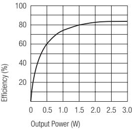
Channel Vo1 (nominal 24V)
