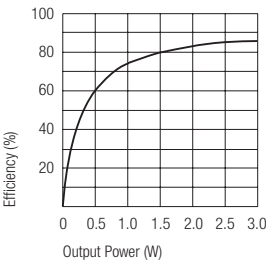
Channel Vo2 (nominal 48V)
