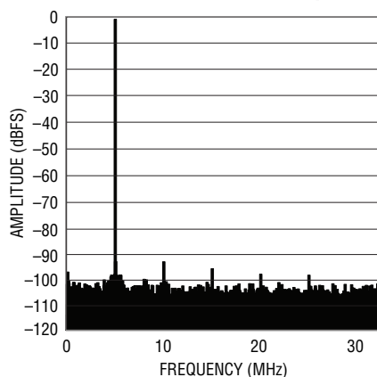
LTC2265-14: 8k Point FFT, f_{IN} = 70\text{MHz} , -1\text{dBFS} , 65\text{Mpsps}
