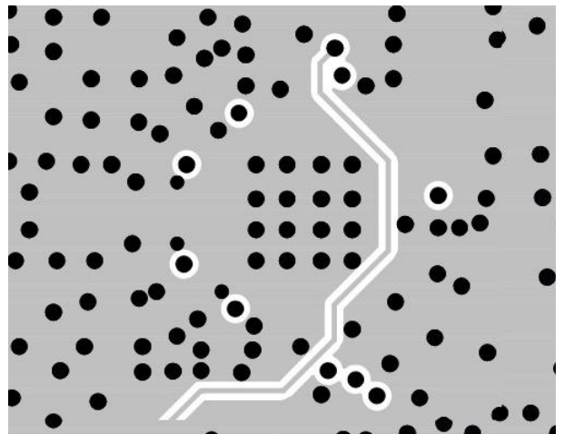
Inner Layer 3
