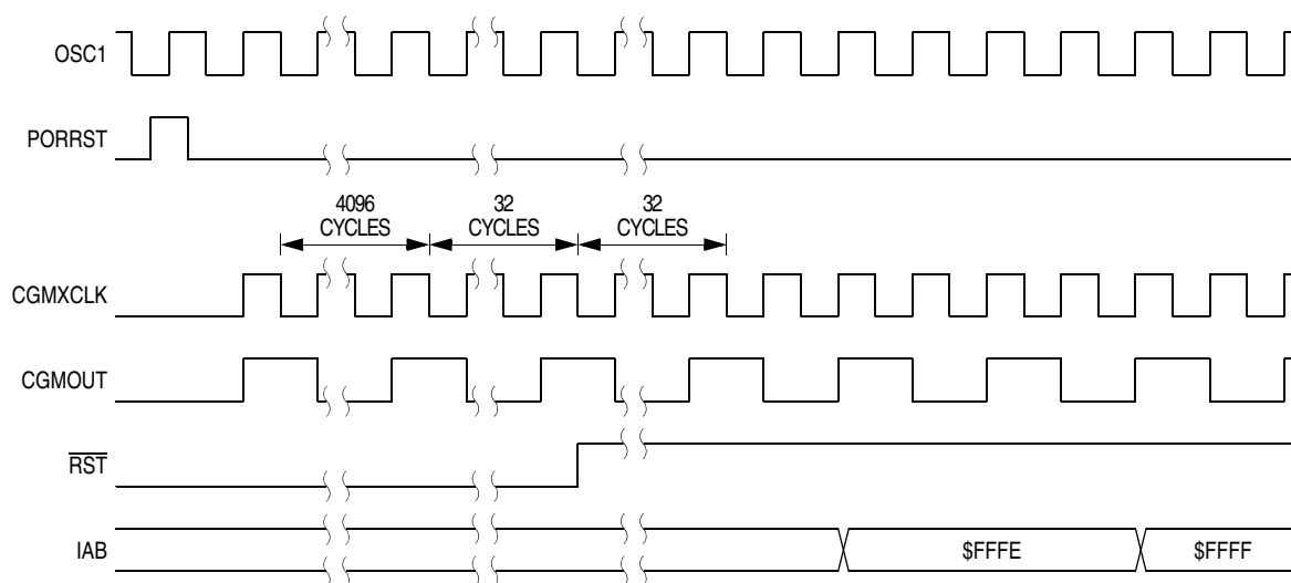
Figure 10-7. POR Recovery
