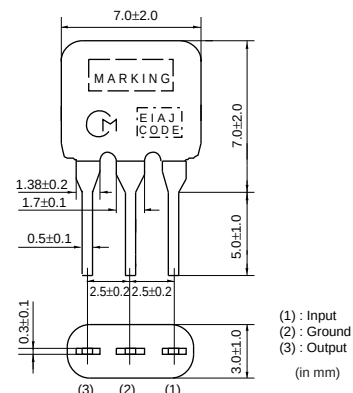
SFELF10M7GALP03-B0
