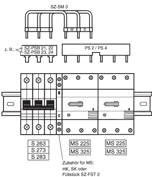
Verbindungsstück SZ-SM3 Einspeisung oben
