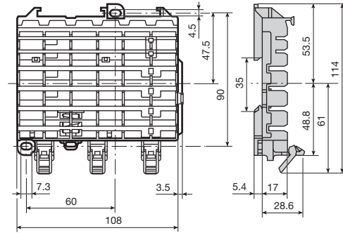
Stecksocket ZLS 806, 6 PLE
