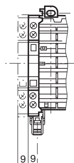
Hilfsschalterblock HK mit Leergehäuse ZLS 930, 1 PLE
