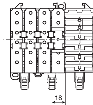
Sammelschienen-Abdeckung ZLS 100 mit Aufbauadapter ZLS 101
