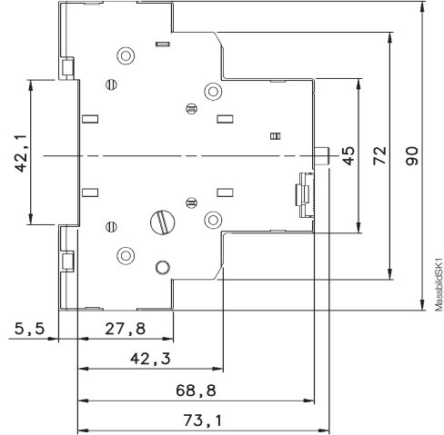
Signalkontakt SK1
