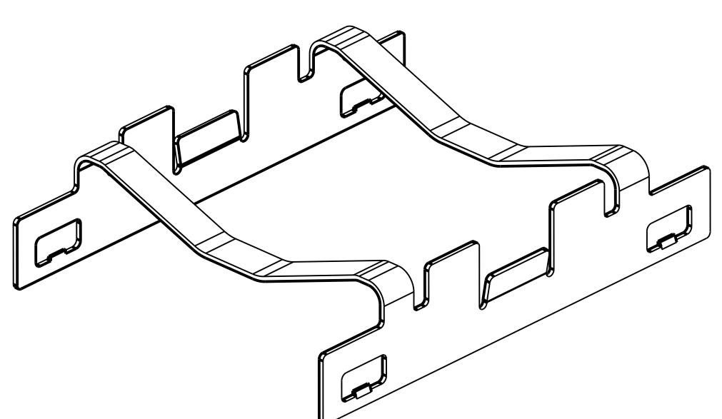
2007304-5 SCALE 4:1
