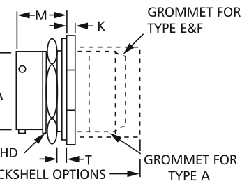
CRIMP KPSE07 (MS3124)
