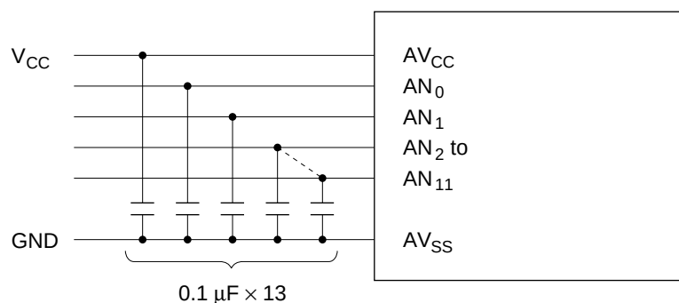
Figure 54 Example of Connections (AV CC to AV SS )
