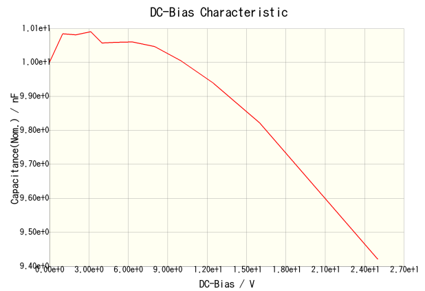
C1608X7R1E103K080AA
