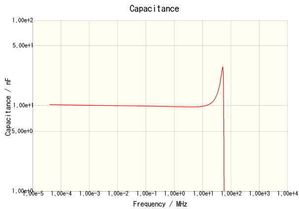
C1608X7R1E103K080AA
