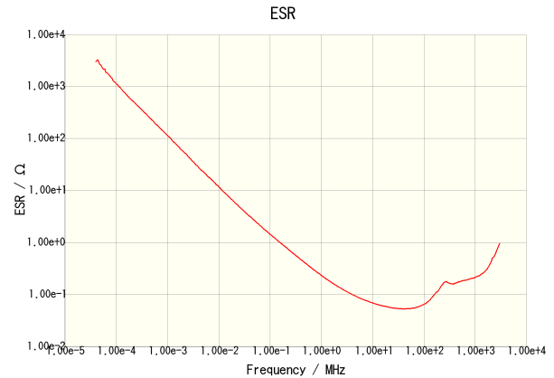
C1608X7R1E103K080AA
