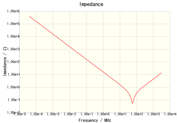
C1608X7R1E103K080AA
