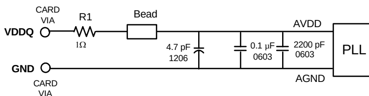
Figure 10. AV DD Filtering [3,4,5]
