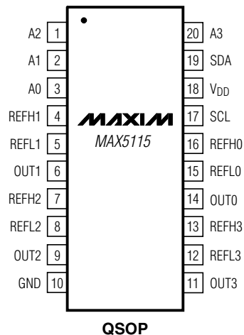
QSOP
