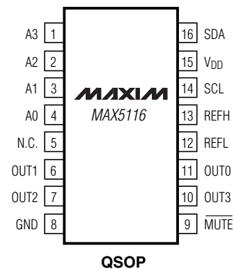
QSOP
