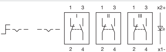
Wiring diagram 279
