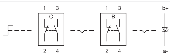
Wiring diagram 285
