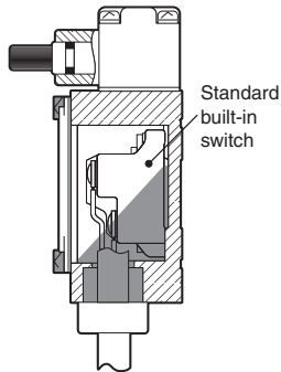
WLG□-145
