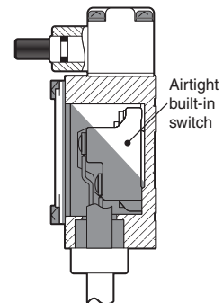
WLG□-RP60 *1
