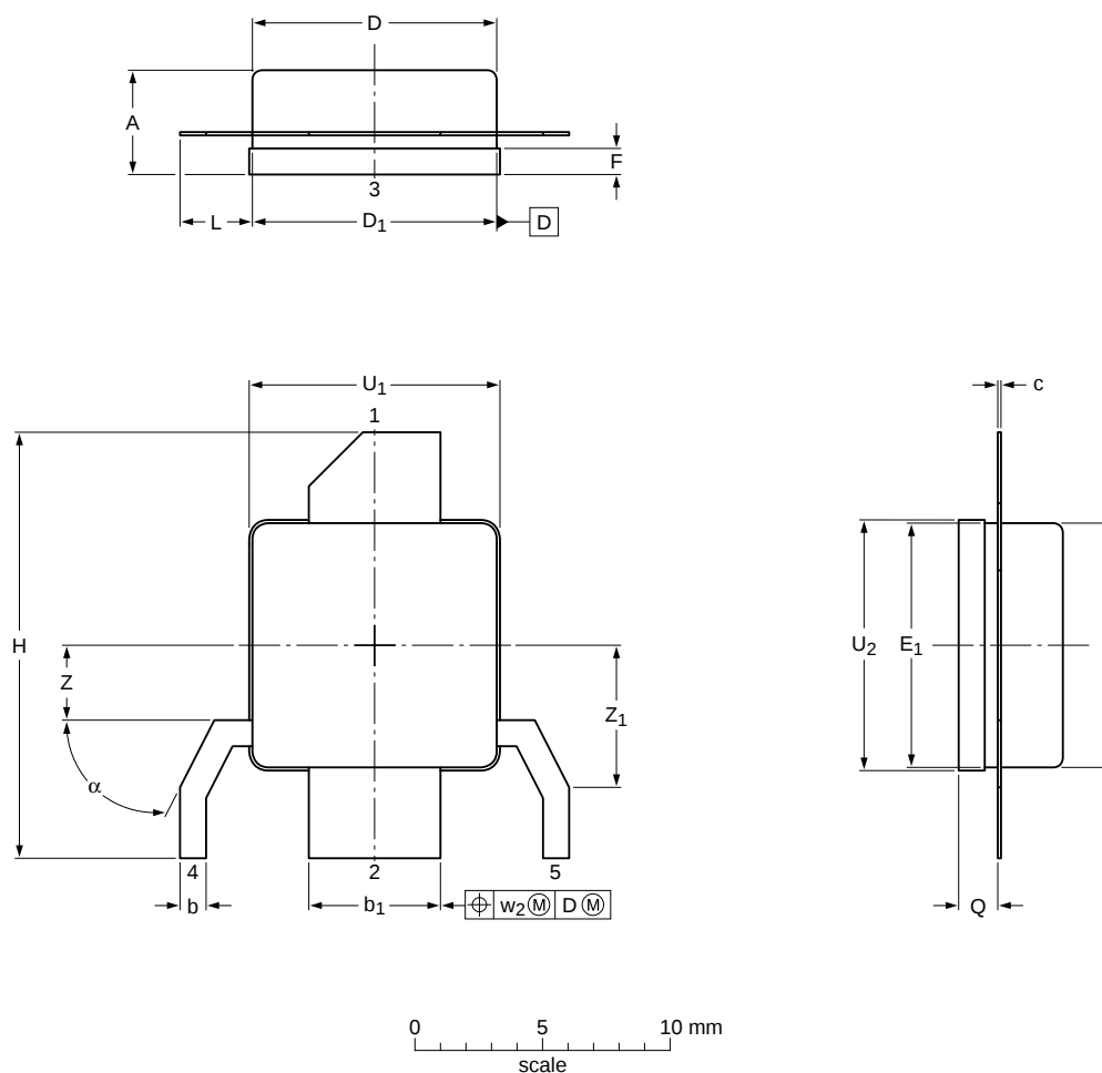
Dimensions
