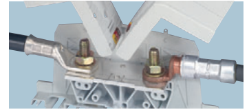
Cable - Cable lug
