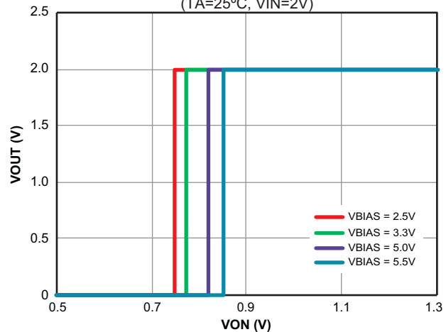
VOUT vs. VON (TA=25°C, VIN=2V)
