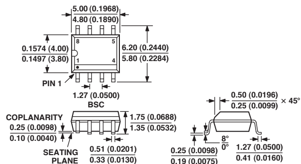
SOIC (R-8)
