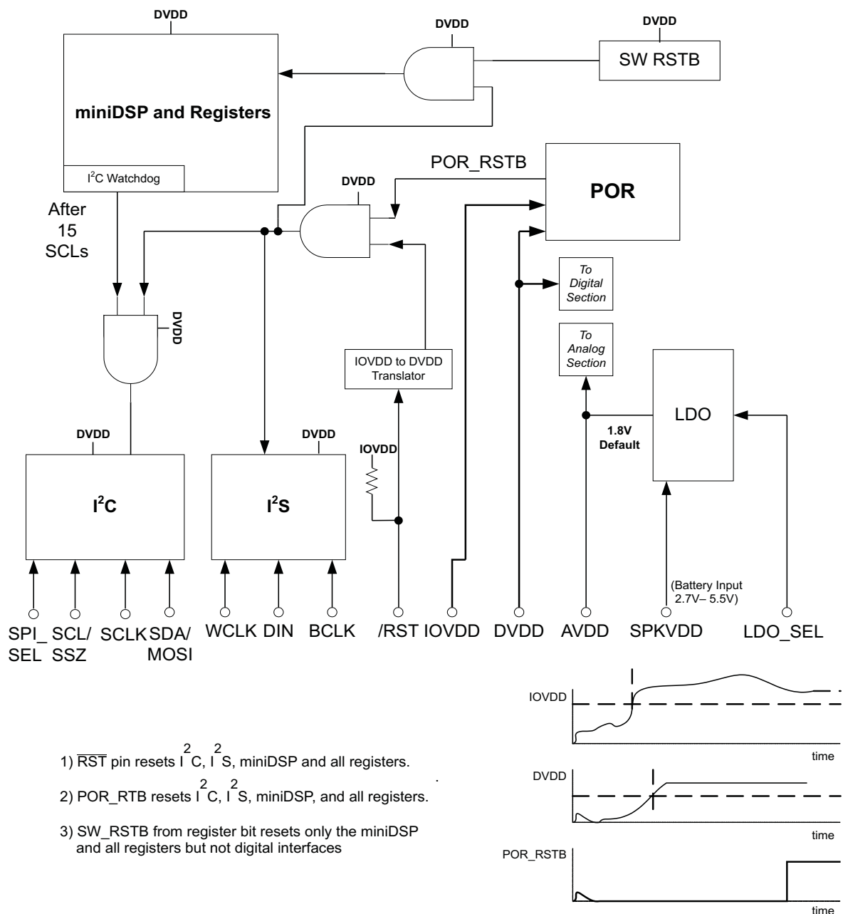
Figure 2-7. POR Diagram
