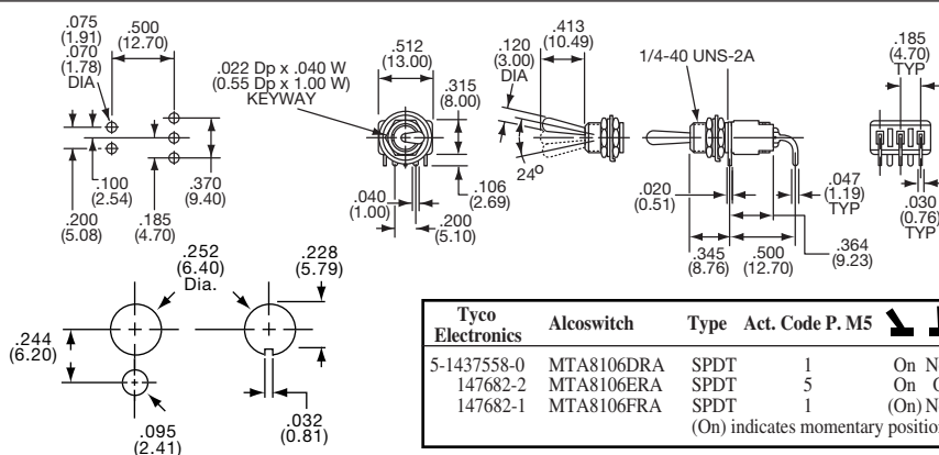
Horizontal Actuation
