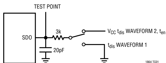
Load Circuit for t_{dPO} , t_r , t_f , t_{dis} and t_{en}
