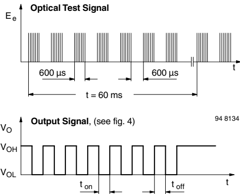
Fig. 3 - Output Function
