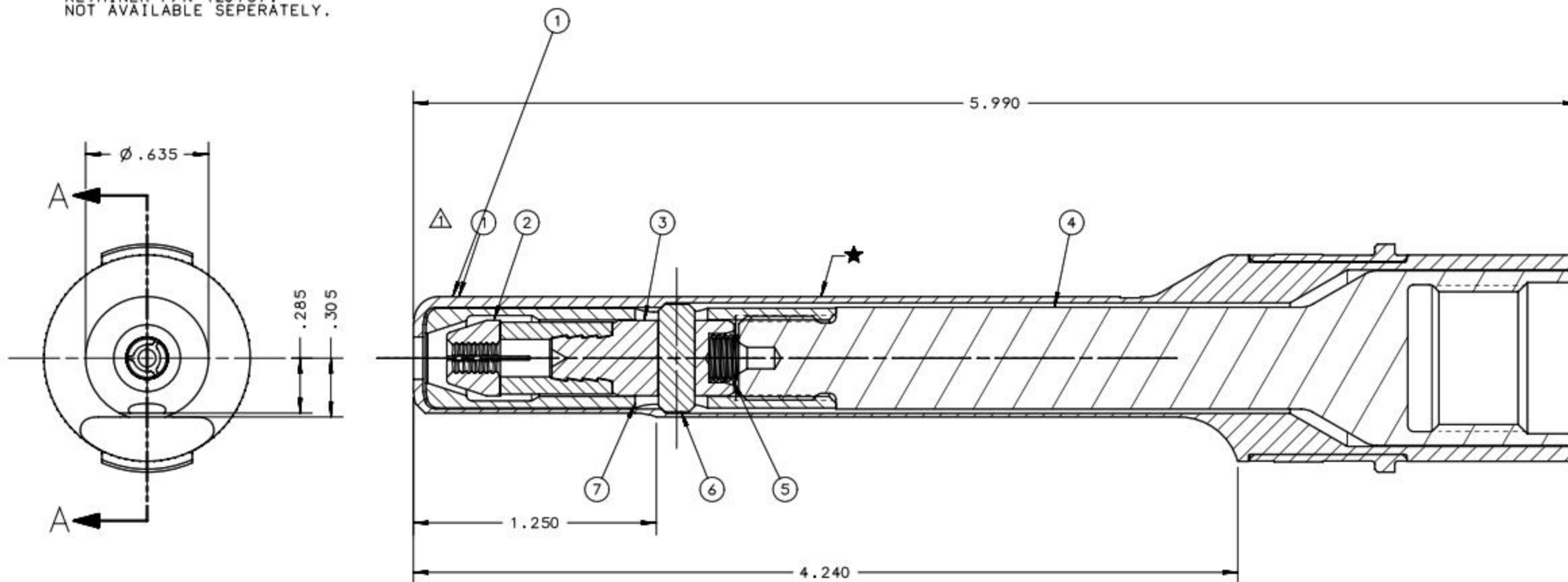
SECTION A-A
