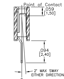
(-02) TOP ENTRY
