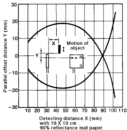
E3C-DS50
