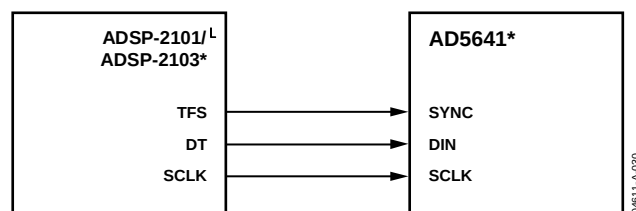
Figure 29. AD5641 to ADSP-2101/ADSP-2103 Interface
