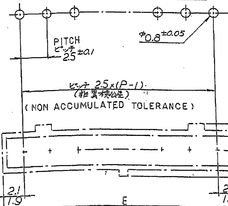
基板加工寸法 FIG.2
