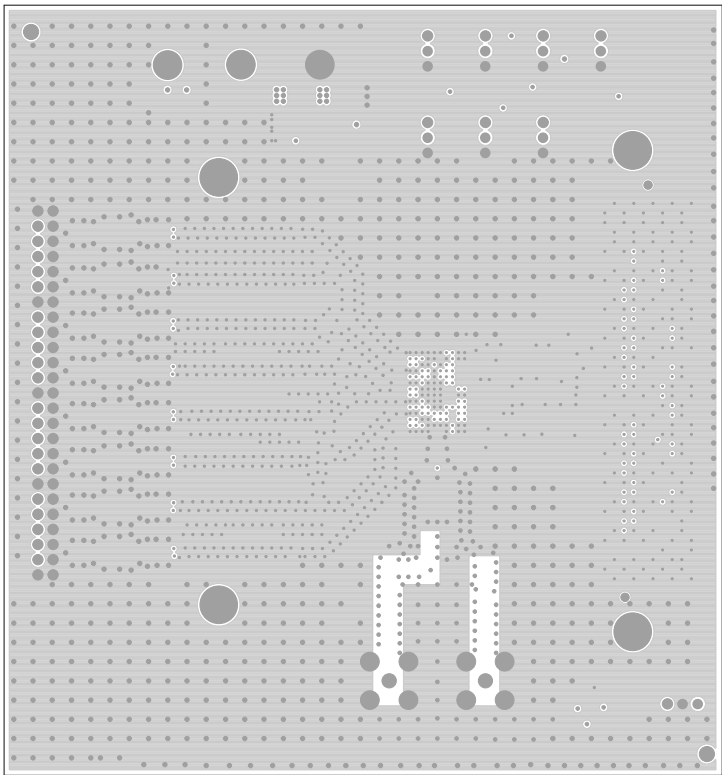
Inner Layer 3
