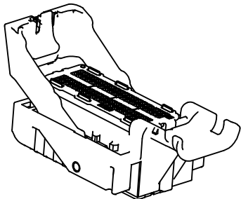
80 CKT SCALE 3:2
