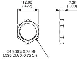
HEX NUT
