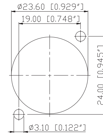
Frontplattenausschnitt (Rückseite) Panel cut out (rear side)
