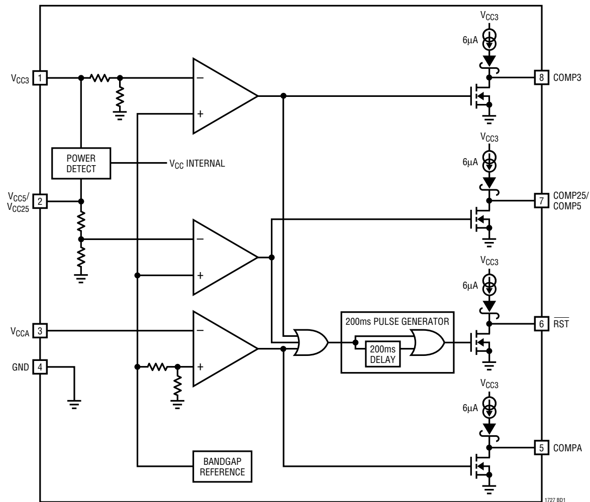
LTC1727-5/LTC1727-2.5
