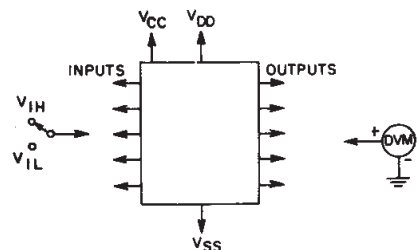
Fig. 8 - Input voltage.
