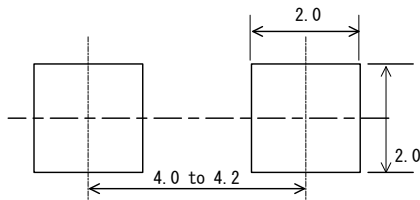
SJP Land Pattern Example
