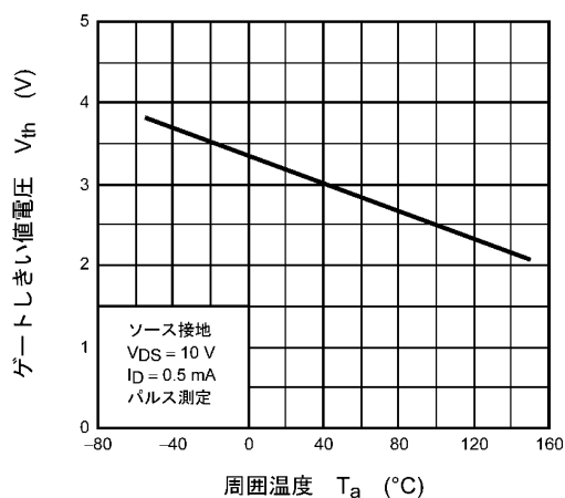
図 8.11 V_{th} - T_a
