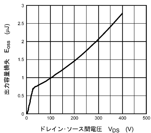
図 8.10 E_{oss} - V_{DS}
