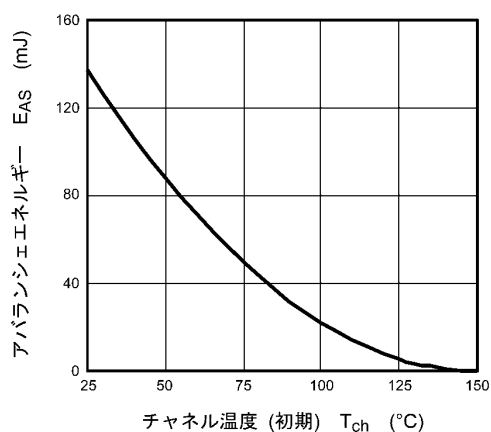
図 8.14 E_{AS} - T_{ch} (最大値 (保証値))
