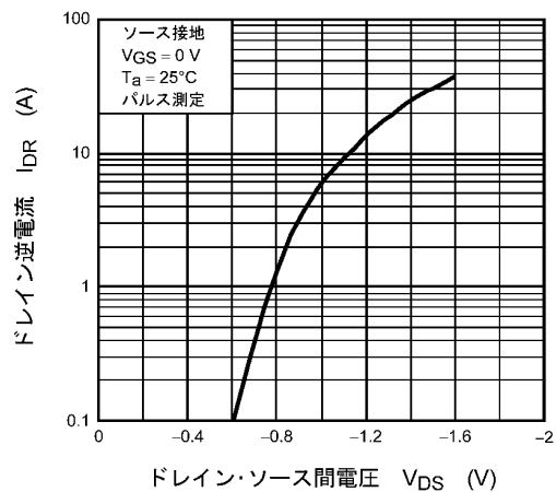
図 8.8 I_{DR} - V_{DS}
