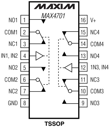
TSSOP
