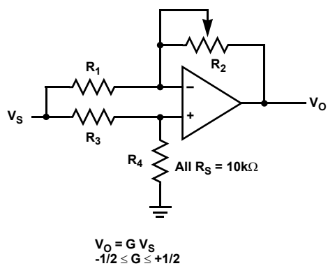
ATTENUATOR
