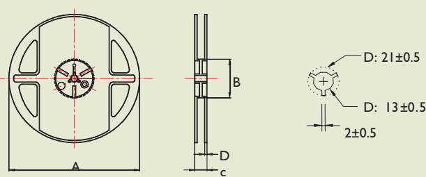
Reel Dimensions
