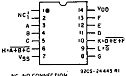
CD4000UB
