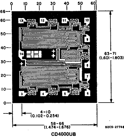
CD4000UB
