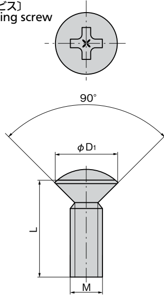
化粧ビス Dressing screw
