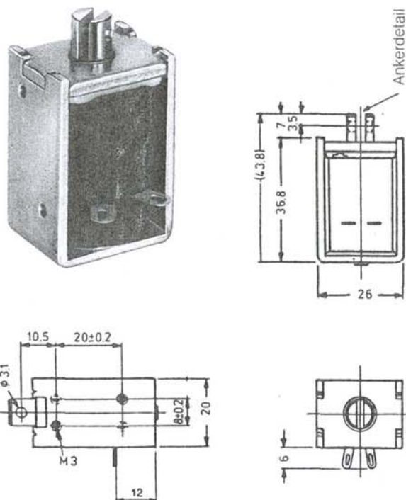
Ankerdetail
