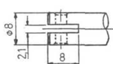
Ankerdetail
