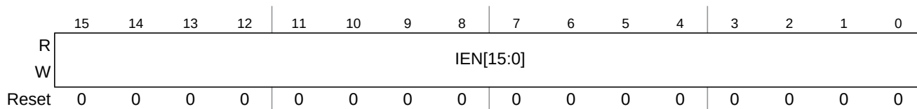
Figure 24-12. ATD Input Enable Register (ATDDIEN)
