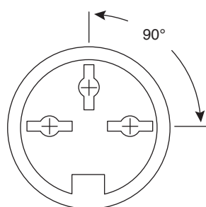
3 Contacts 161-0003-E
