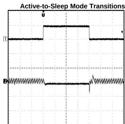
V_{IN} = 3.6V , V_{OUT} = 1.5V , Load = 20mA CH1: SLEEP pin; Scale: 2V/Div CH2: V_{OUT} ; Scale: 200mV/Div Time scale: 200µs/Div
