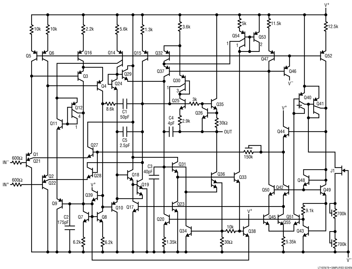
1/2 LT1078, 1/4 LT1079
