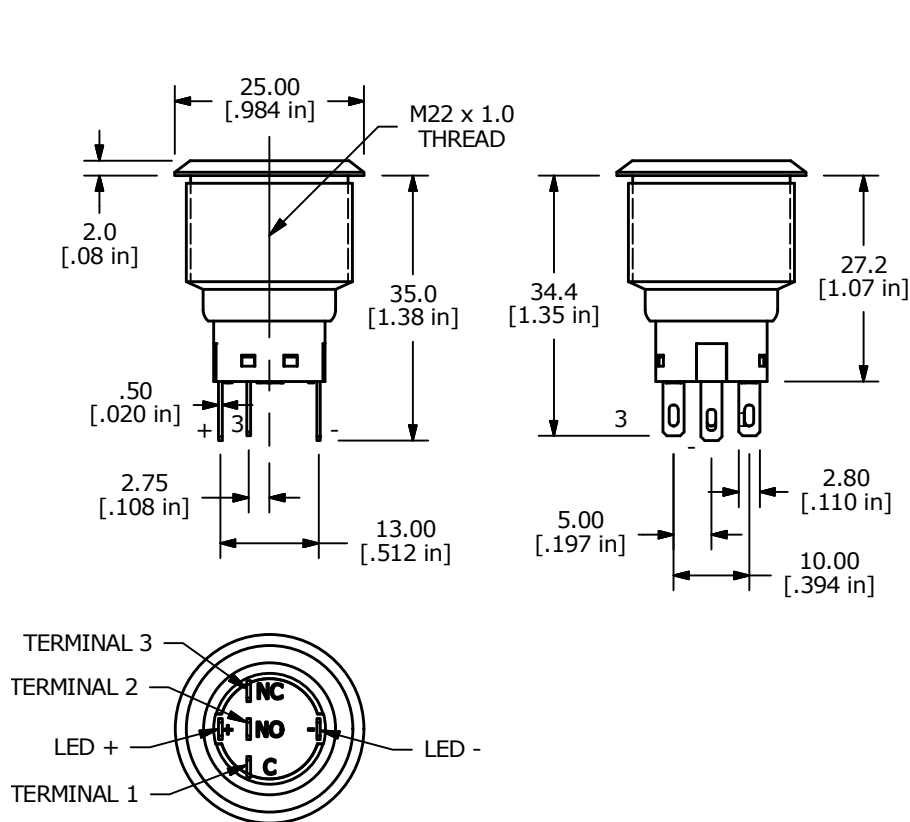
SPDT SWITCH DIMENSIONS
